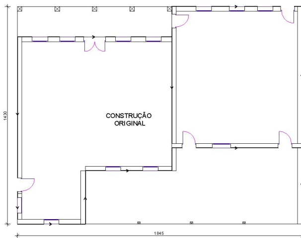
PLANTA BAIXA
